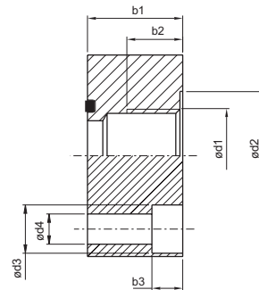
B.S.P.P. flange
